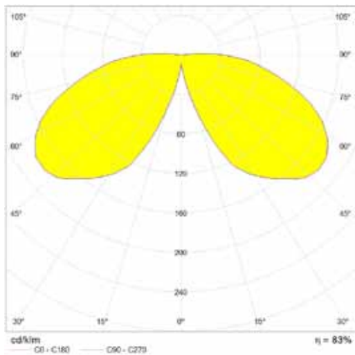
Afbeelding 3: NU-Led Polar Curve
